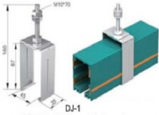
DJ-1 M10 Sürgülu Kayar Askı Aparatı
